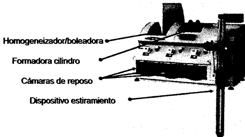
Figura 11: Extensografo Brabender.
