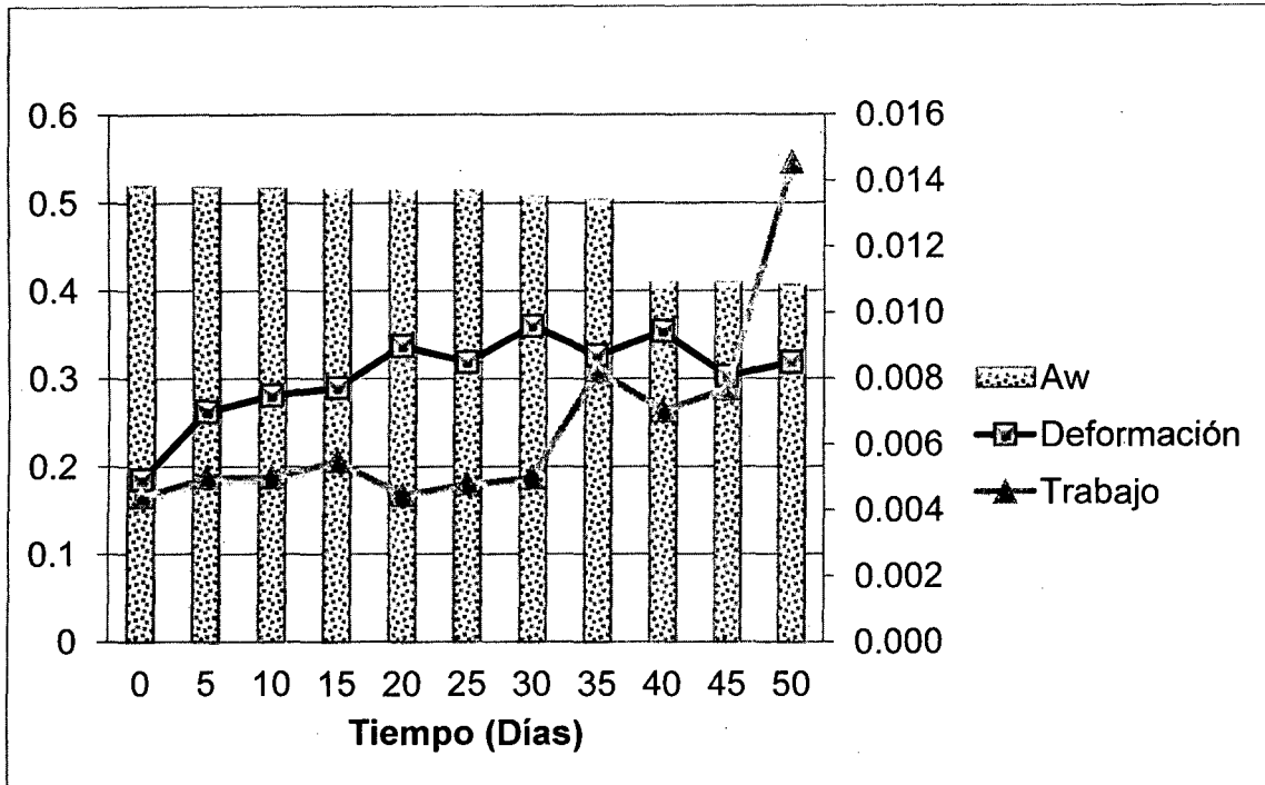
GRÁFICO N°04: RESISTENCIA A LA RUPTURA EN FUNCIÓN DE A_w EN LAS BARRAS ENERGÉTICAS
